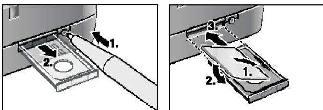
Рисунок 2 Подключение SIM-карты
