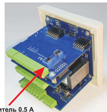
Предохранитель 0.5 А
