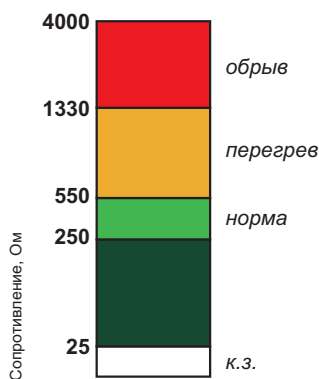
Характеристика РТС-термистора
